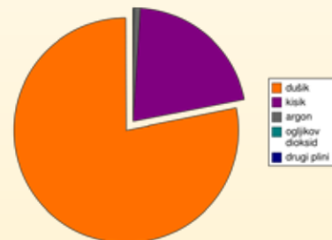
http://sl.wikipedia.org/wiki/Slika:Composition_of_Earth%27s_atmosphere.svg
